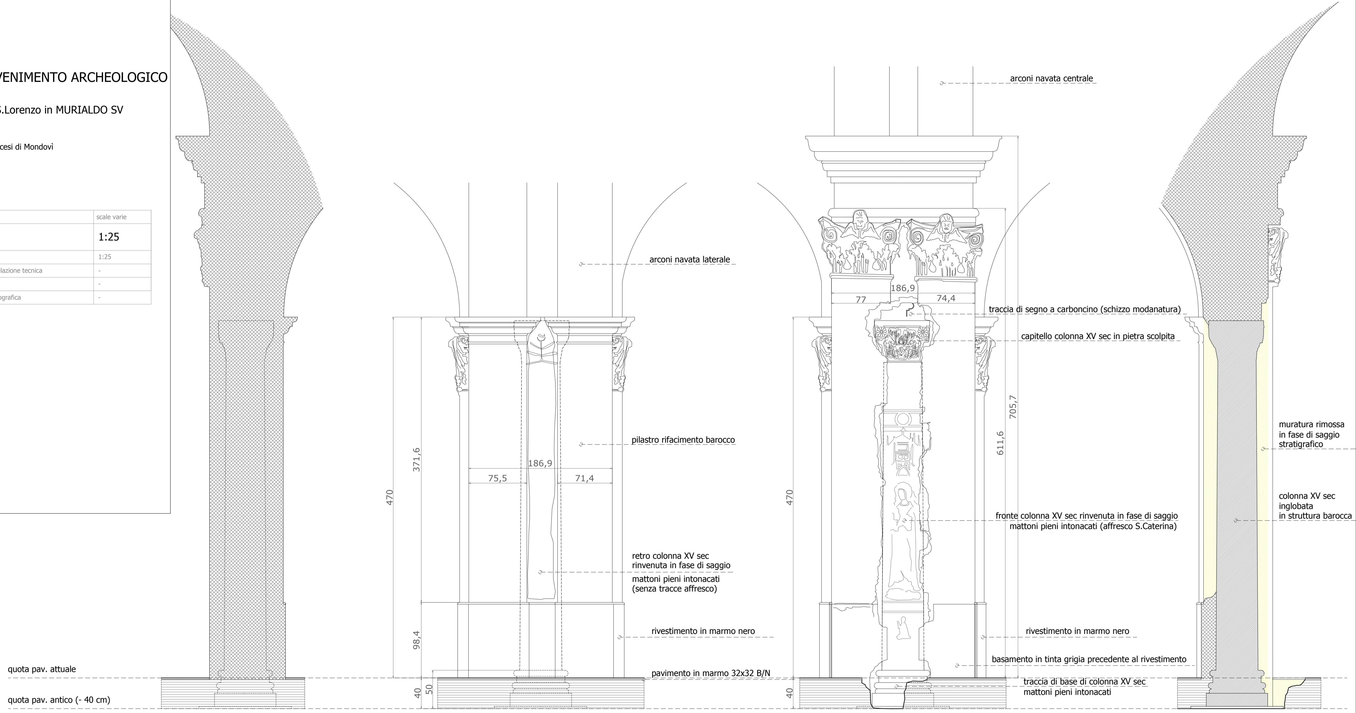
SEZIONE 4 (sezione trasversale su pilastro barocco)
